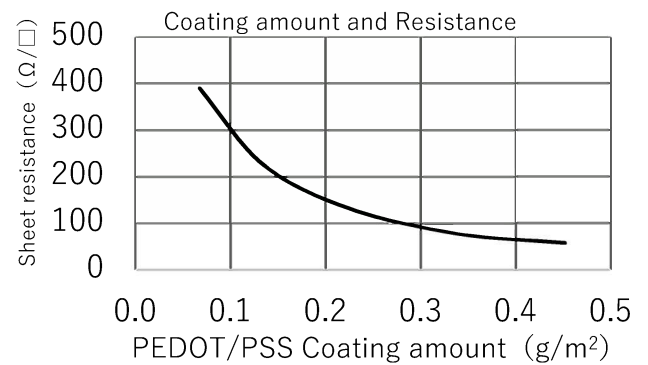
塗布量と抵抗値の関係
