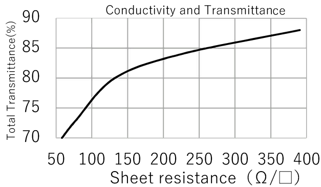
抵抗値と透過率*3の関係
